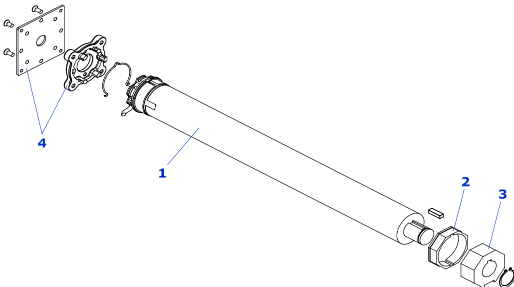
Рисунок 8. Монтаж приводов серии AM2
