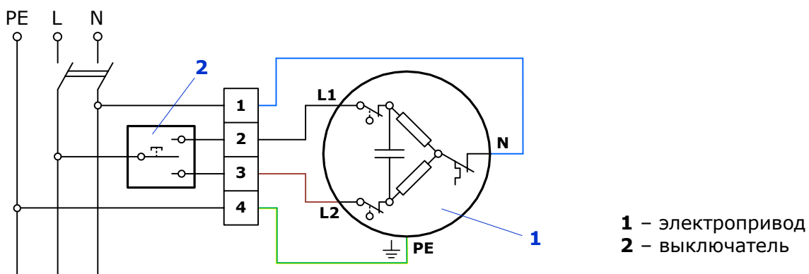
Рисунок 11. Электрические подключения
